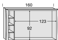
CON LIBRERIA A SX WITH LH BOOKCASE
