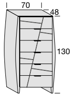
APERTURA CON MANIGLIE OPENING WITH HANDLES
