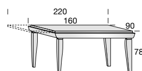
TAVOLO RETTANGOLARE ALLUNGABILE RECTANGULAR EXTENDING TABLE
