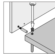
MONTAGGIO PIEDE REGOLATORE ADJUSTABLE FOOT ASSEMBLY
