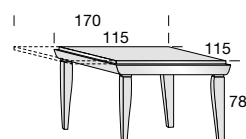
TAVOLO QUADRATO ALLUNGABILE SQUARE EXTENDING TABLE
