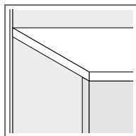
RIPIANI STRUTTURALI A GIORNO SP. 3 - P. 38.2 OPEN STRUCTURAL SHELVES TH. 3 - D. 38.2
