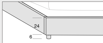
GIROLETTO LEGNO IN PANNELLO LISTELLARE FRASSINO PIEDE IN PLASTICA H. 6 CM
